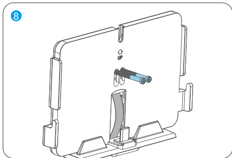
10. 장착 베이스의 위치를 조정하고 나사를 조입니다.
